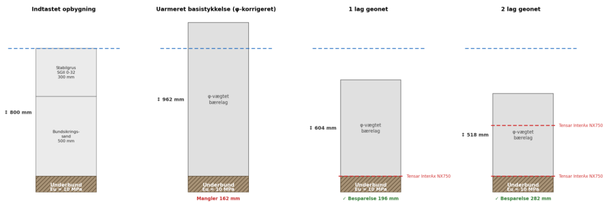
Designndiagram — E_o = 120 \text{ MN/m}^2 · Klasse 5 Materialer: \phi = 36,9^\circ · Geonet: Tensar InterAx NX750
