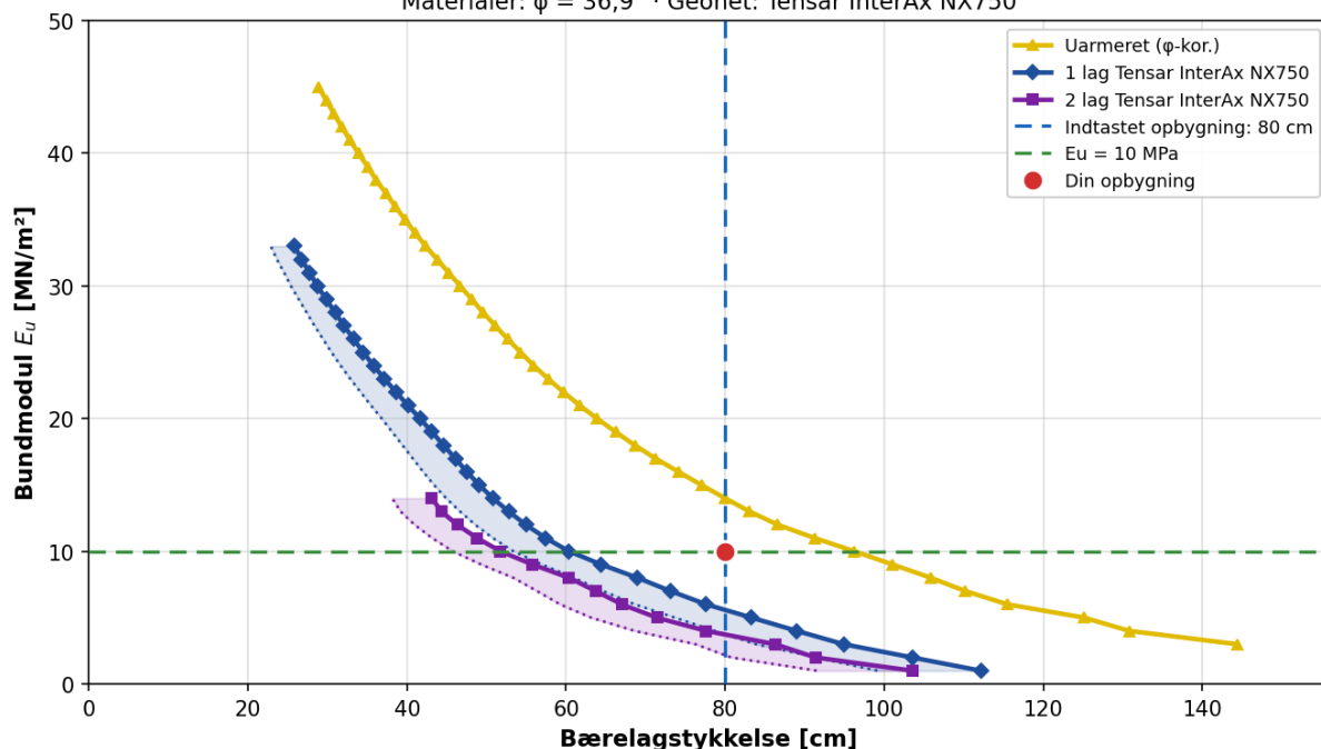
Designndiagram — E_o = 120 \text{ MN/m}^2 · Klasse 5 Materialer: \phi = 36,9^\circ · Geonet: Tensar InterAx NX750
